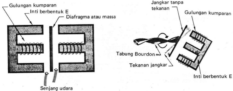
(a) Induktor Kumparan Ganda
