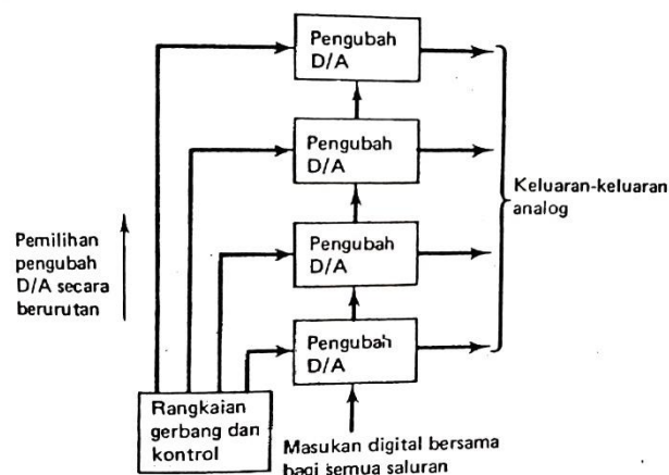
Gambar 3.13. Multiplekser DAC menggunakan beberapa pengubah
