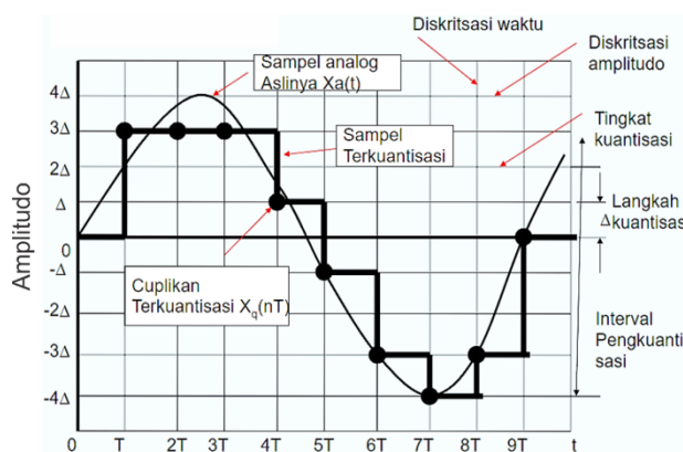
Gambar 3.11. Kuantisasi sinyal sinusoida
