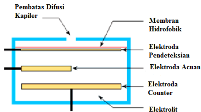
Gambar 0.53 Sensor Gas Elektrokimia
