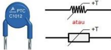
Gambar 0.20 Bentuk Fisik dan Simbol PTC
