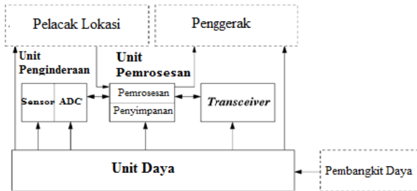
Gambar 0.1 Arsitektur Node Sensor
