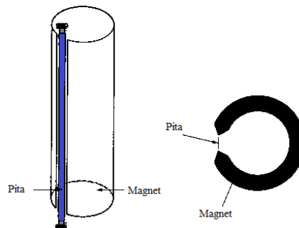
Gambar 0.37 Mikrofon Pita
