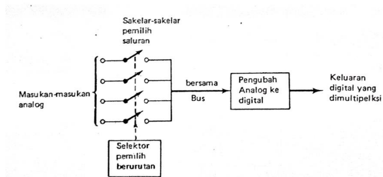
Gambar 3.15. Sistem konversi ADC yang termultiplexsi (Sumber: William DC, 1985)
