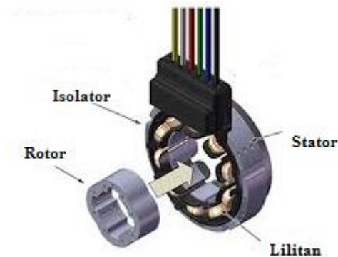
Gambar 0.14 Konfigurasi Resolver
