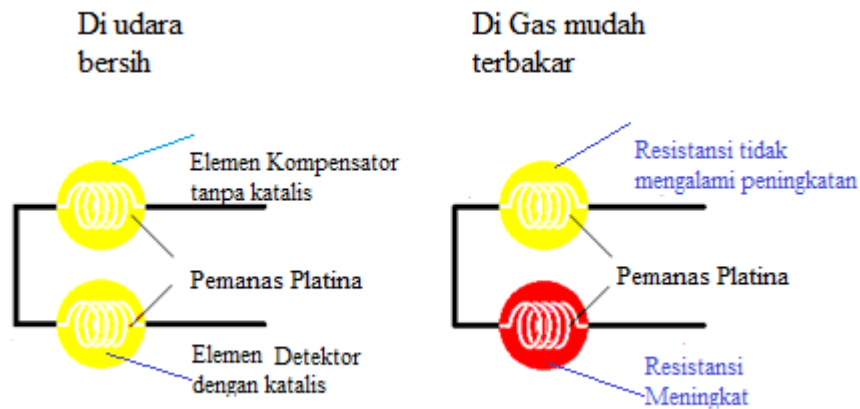
Gambar 0.52 Sensor Gas Katalitik
