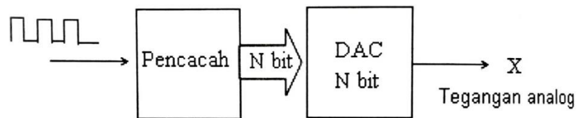
Gambar 3.4. Simulasi konversi DAC
