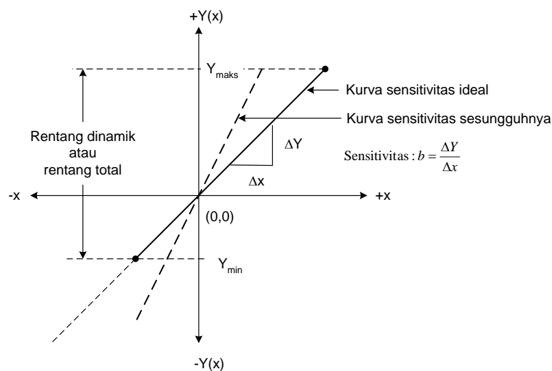
Gambar 2.1 Kurva sensitivitas
