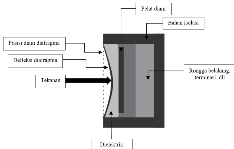
Gambar 2.1. Transduser kapasitif
