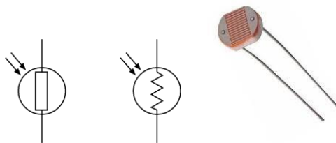
Gambar 0.27 Detektor Fotokonduktif
