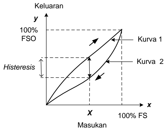
Gambar 2.6. Kurva histeresis
