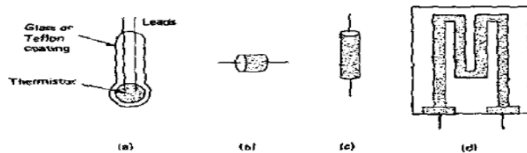
Gambar 0.18 Konfigurasi Termistor
