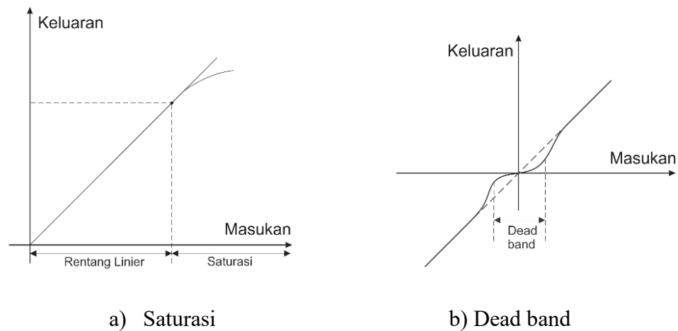
Gambar 2. 5 Kurva saturasi dan kurva dead band
