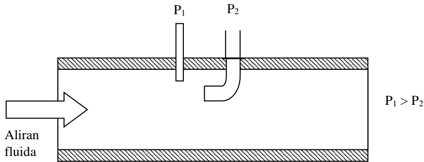
Gambar 0.46 Tabung Pitot
