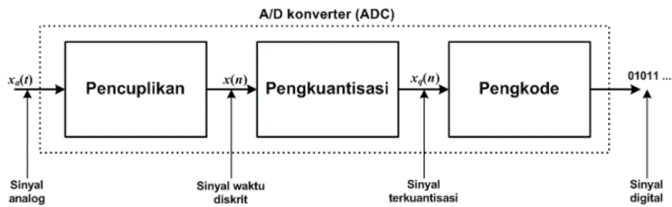
Gambar 3.9. Langkah-langkah ADC (Sumber: Indrasary, 2016)
