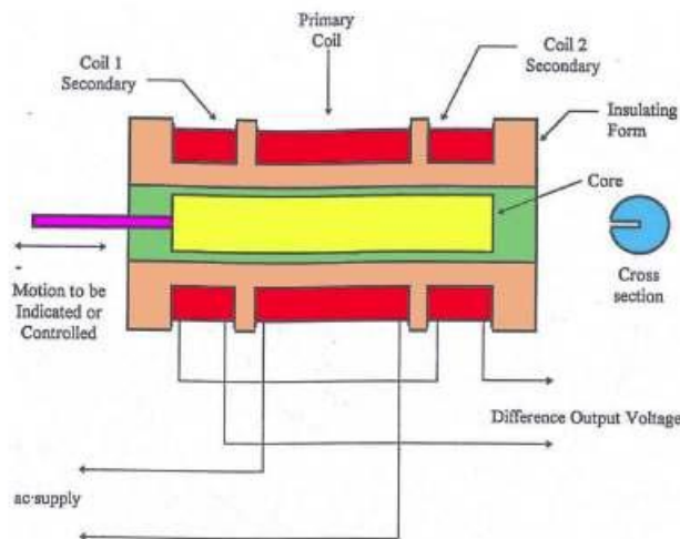
Gambar 0.4 Ilustrasi LVDT
